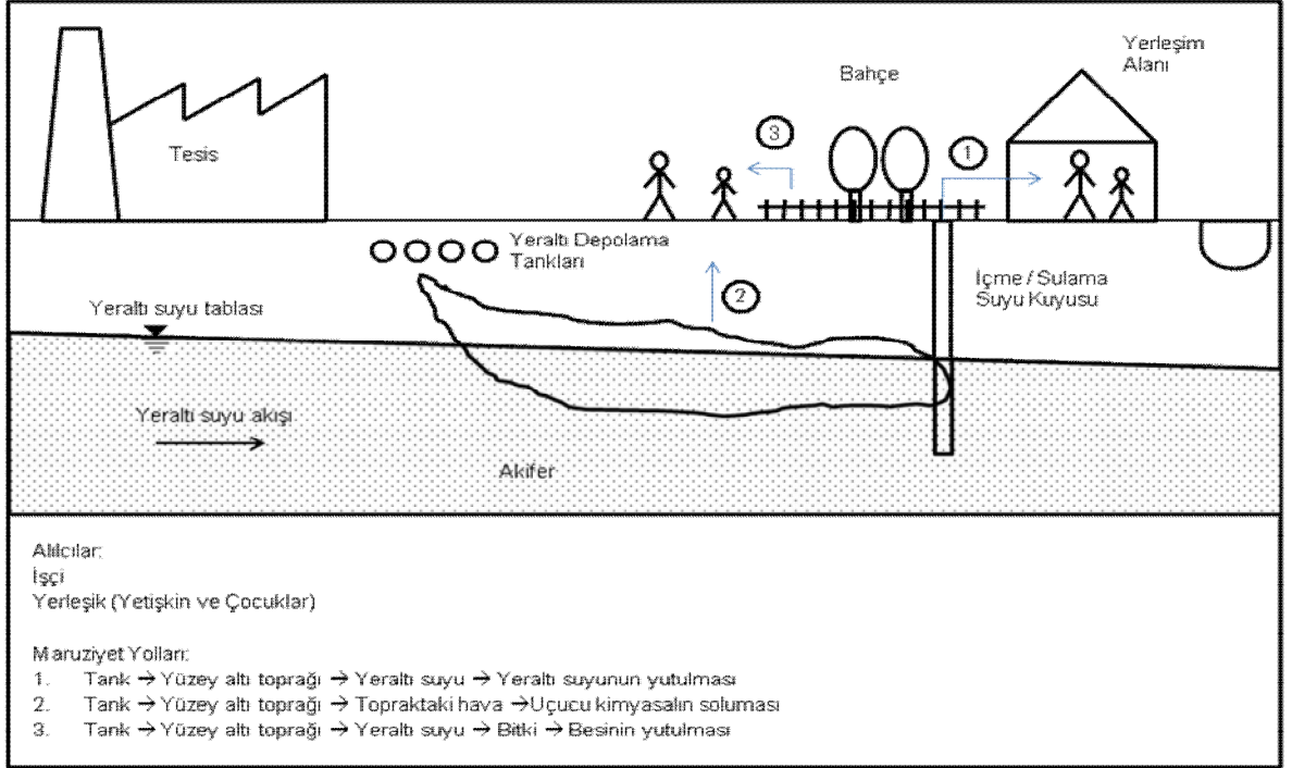
Şekil 3.2. Örnek KSM Şeması – Yan kesit
