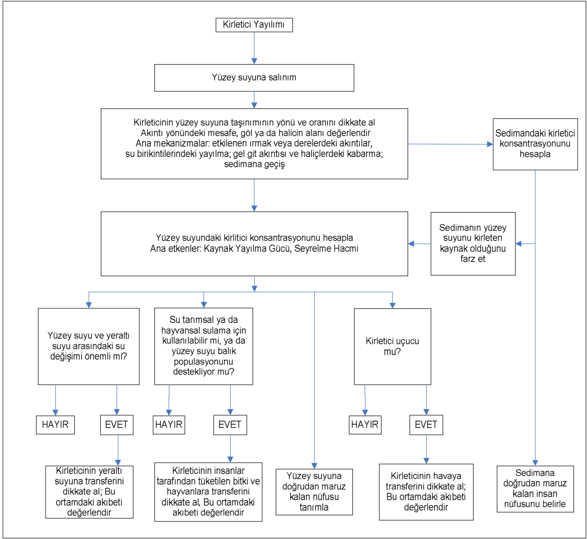
Şekil 5.2. Kirleticilerin Çevresel Ortamlardaki Davranışlarının ve Taşınımlarının Değerlendirilmesinde Kullanılacak Akım Şeması: Yüzey Suyu ve Sediman (U.S. EPA, 1989)
